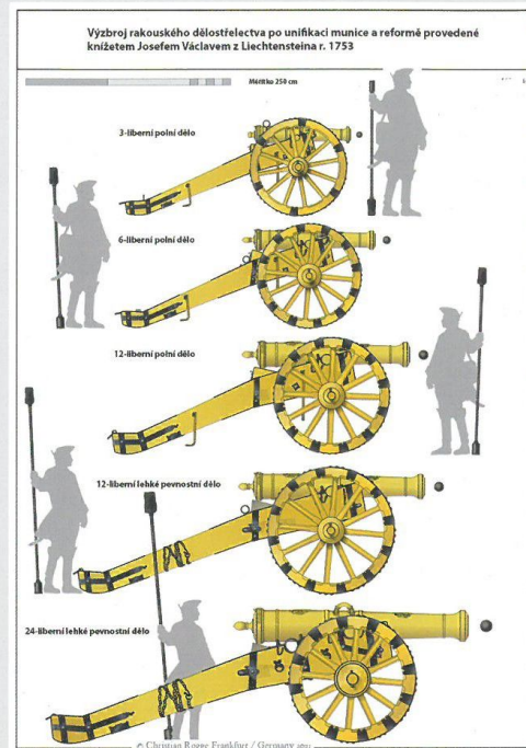
Typologie rakouských polních a pevnostních děl po reformaci rakouského dělostřelctva provedené Josefem Václavem knížetem z Liechtenštejna v roce 1753
